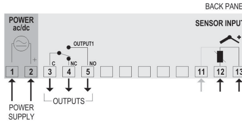
Fig. 1 - N321 terminals
