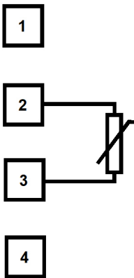
2 Wire
