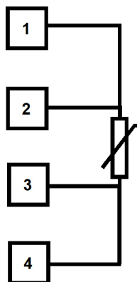
4 Wire
